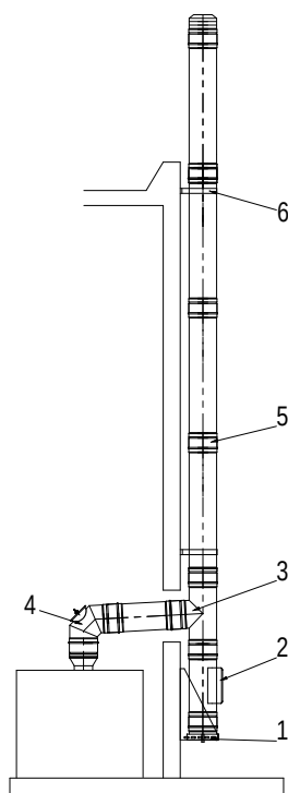
Bild 17: Montagebeispiele
