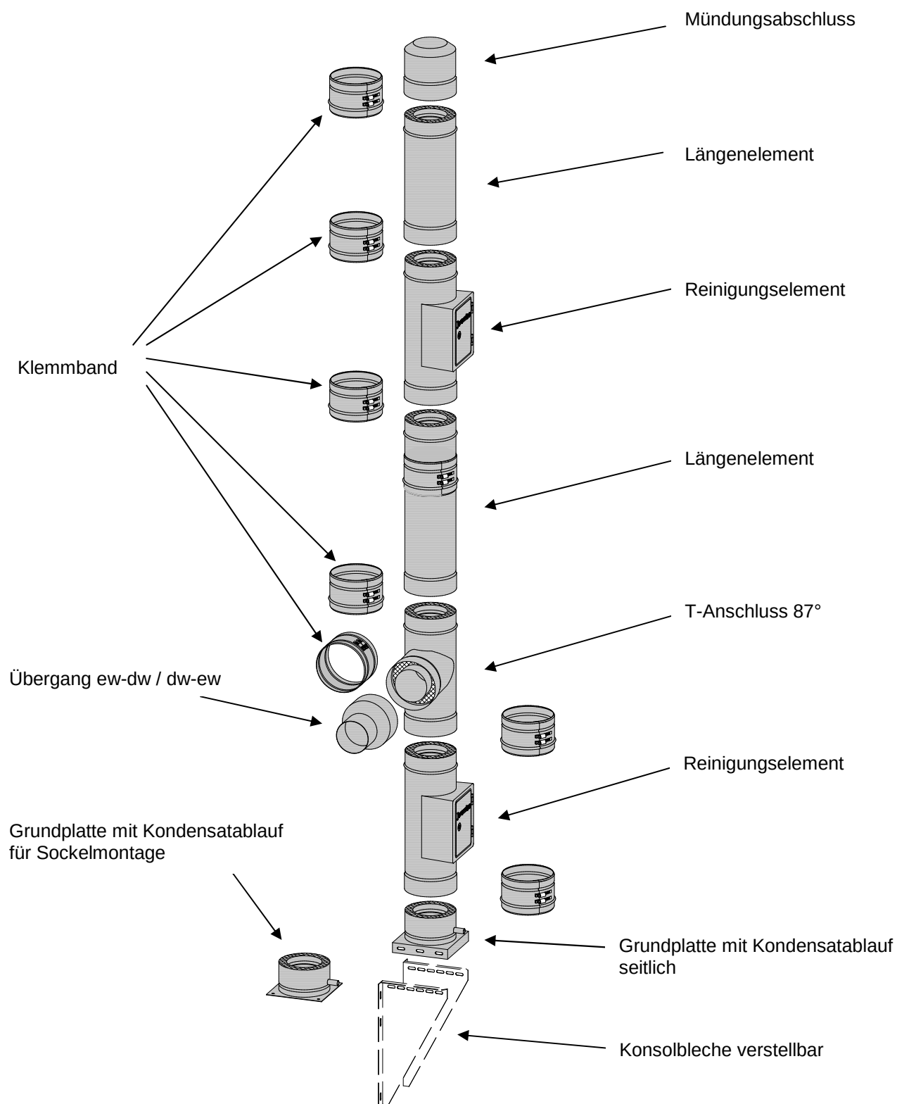
Bild 18: Bauteilübersicht
