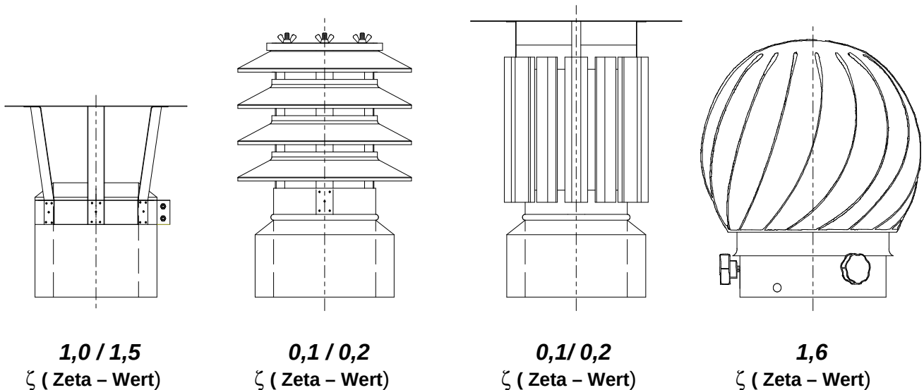
Bild 16: Aufsätze
