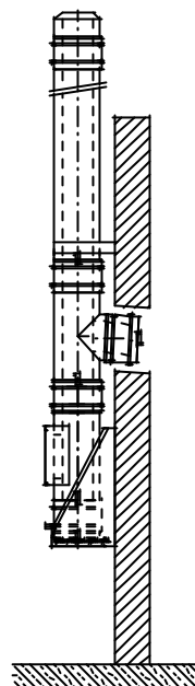
Bild 4: Aufbau Grundplatte mit Kondensatablauf und Konsolblech nach oben
