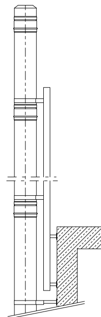
Bild 12: Aufbau mit Kragarm
