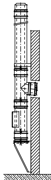
Bild 5: Aufbau Grundplatte mit Kondensatablauf und Konsolblech nach unten
