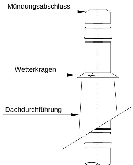
Bild 11: Dachdurchführung
